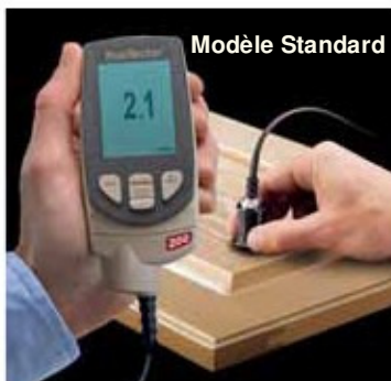
Sonde B mesure de revêtements polymères sur bois, plastique, etc.
